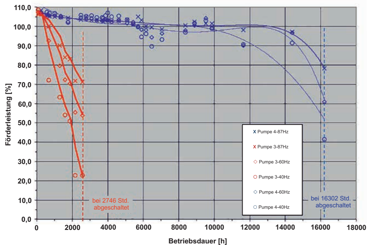
Förderleistung = f (Betriebsdauer)
